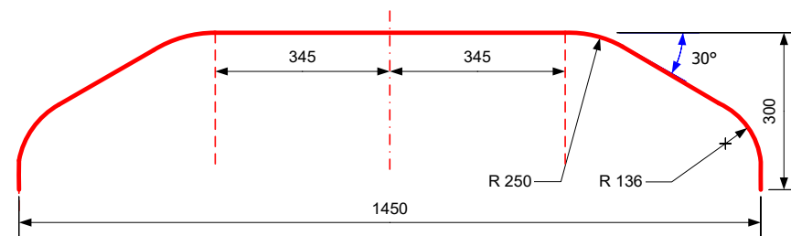
Slika 3 – Profil glave oduzimača struje za kontaktnu mrežu 3 kV (3R120)
