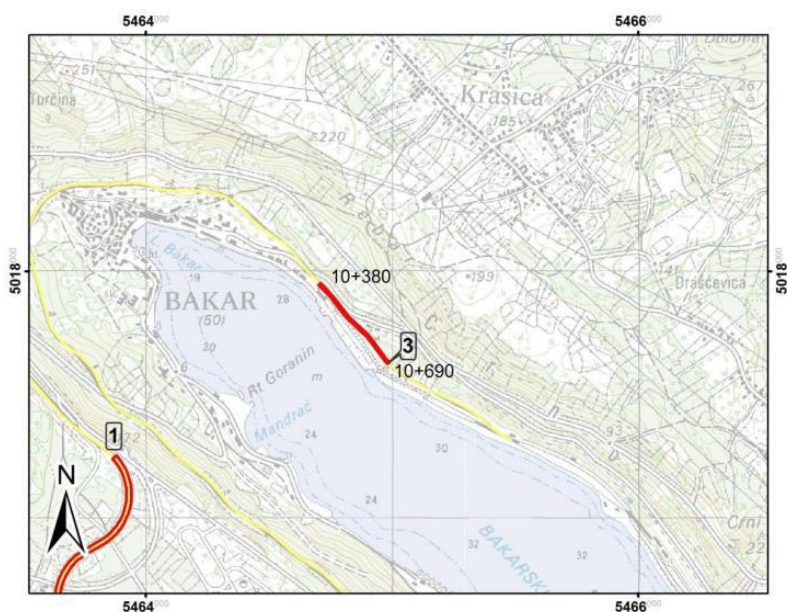
Slika 2. Topografski prikaz usjeka Bakar, pruga M 602 Škrljevo- Bakar, dionica Šoići – Bakar
